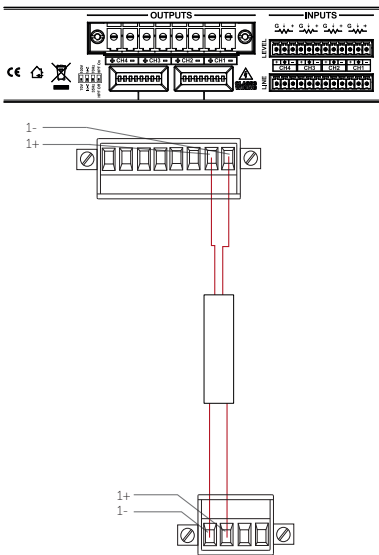
Figure 4.7: Bias Q1/Q1.5/Q2 Phoenix wiring
