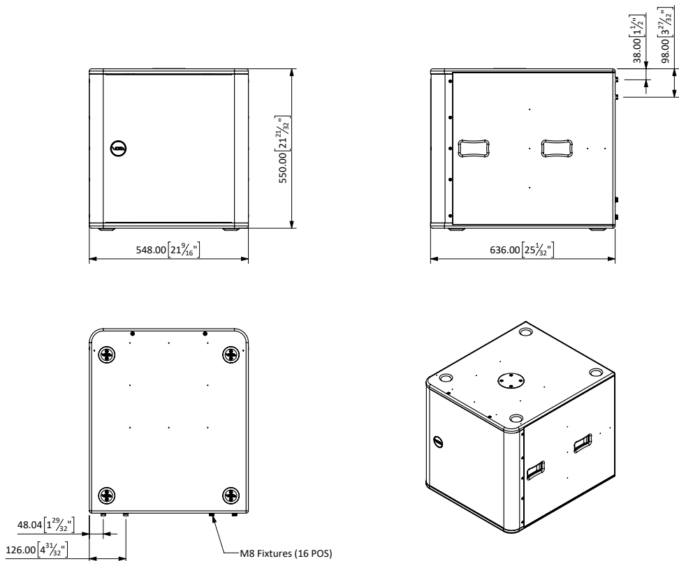
Figure B.11: Venu 118 V2 dimensions
