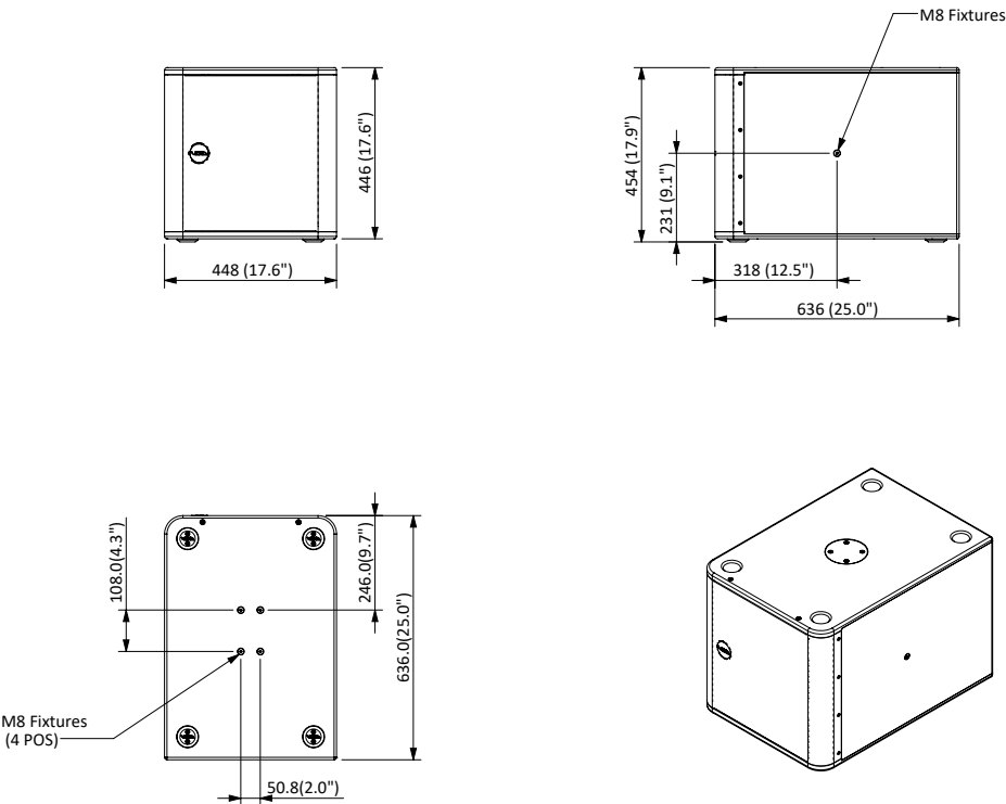
Figure B.9: Venu 115 V2 dimensions
