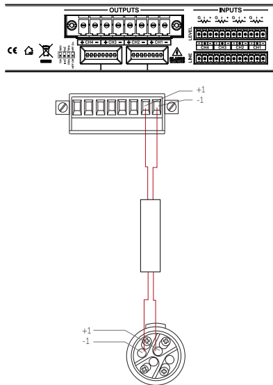
Figure 4.10: Bias Q1/Q1.5/Q2 Phoenix wiring
